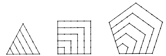
Dreieckszahlen 1, 1+2=3, 1+2+3=6, ... Viereckszahlen 1, 1+3=4, 1+3+5=9, ... Fünfeckszahlen 1, 1+4=5, 1+4+7=12, ...
